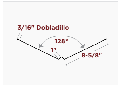
VALLE FORMADO ESTILO W DE 20" CON DOBLADILLOS DE 10'
