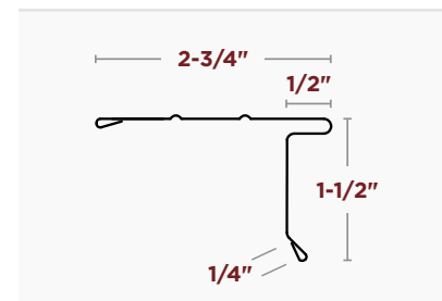
BORDE DE TECHO ESTILO SR de 5"
