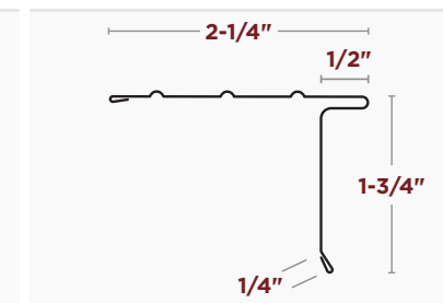
BORDE DE TECHO ESTILO SRLF de 5"
