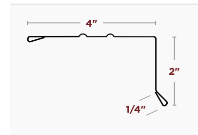
BORDE DE TECHO ESTILO A de 2"X4"
