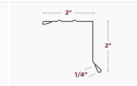
BORDE DE TECHO ESTILO A de 2"X2"
