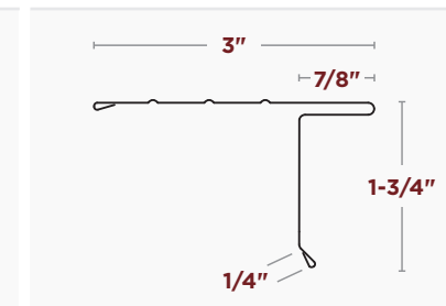
BORDE DE TECHO ESTILO L de 6"
