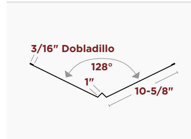
VALLE FORMADO ESTILO W DE 24" CON DOBLADILLOS DE 10'
