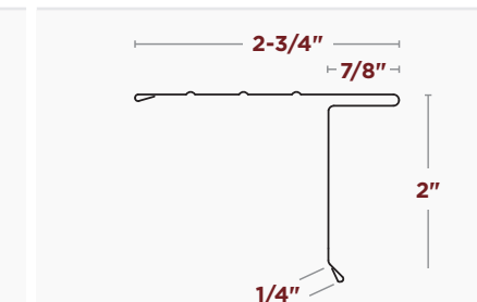
BORDE DE TECHO ESTILO LL de 6"
