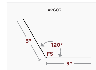
TAPAJUNTAS DE ÁNGULO INTERIOR DE 4"x5" (120 GRADOS)
