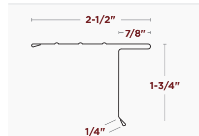
BORDE DE TECHO ESTILO L de 5-1/2"
