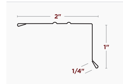
BORDE DE TECHO ESTILO A de 1"X2"
