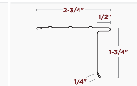
BORDE DE TECHO ESTILO SRLF de 5-1/2"
