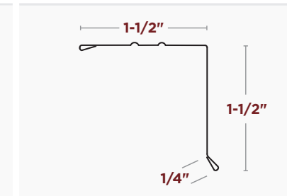
BORDE DE TECHO ESTILO A de 1-1/2"X1-1/2" (DISPONIBLE CON GRABADO EN RELIEVE)
