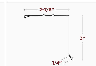
BORDE DE TECHO ESTILO A de 3"X3"
