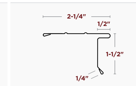
BORDE DE TECHO ESTILO SR de 4-1/2"
